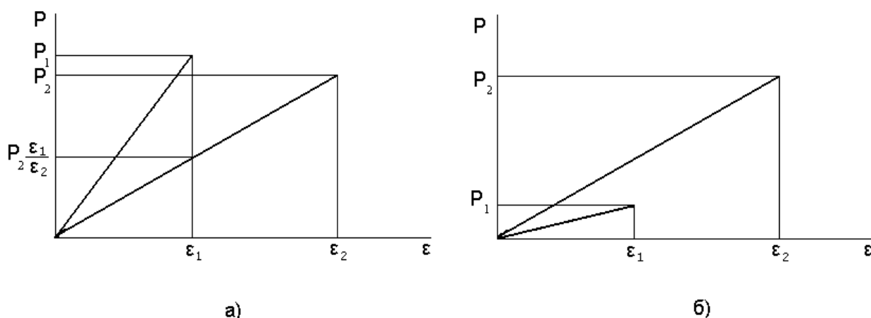
Рисунок 3 - Кривые растяжения компонентов армированной нити при условии: а) P_{РАЗР} > P_2 ; б) P_{РАЗР} \leq P_2
