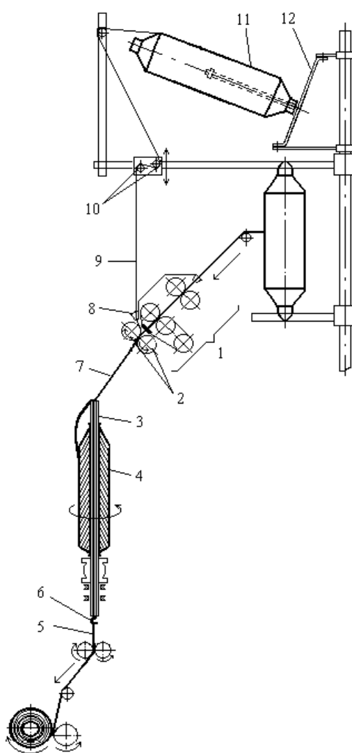
Рисунок 2 – Технологическая схема модернизированной прядильно-крутильной машины для производства комбинированных швейных ниток
